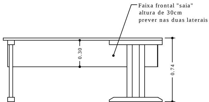
Elevação
