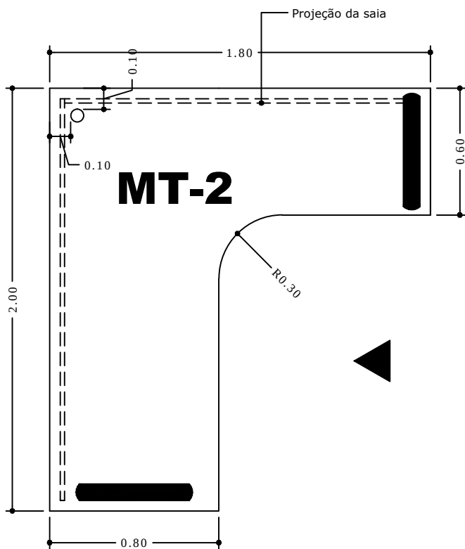
Planta
