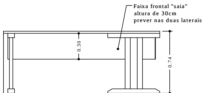
Elevação
