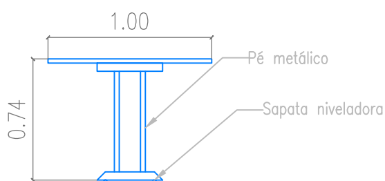
Vista lateral
