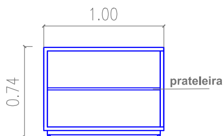
Vista frontal sem portas
