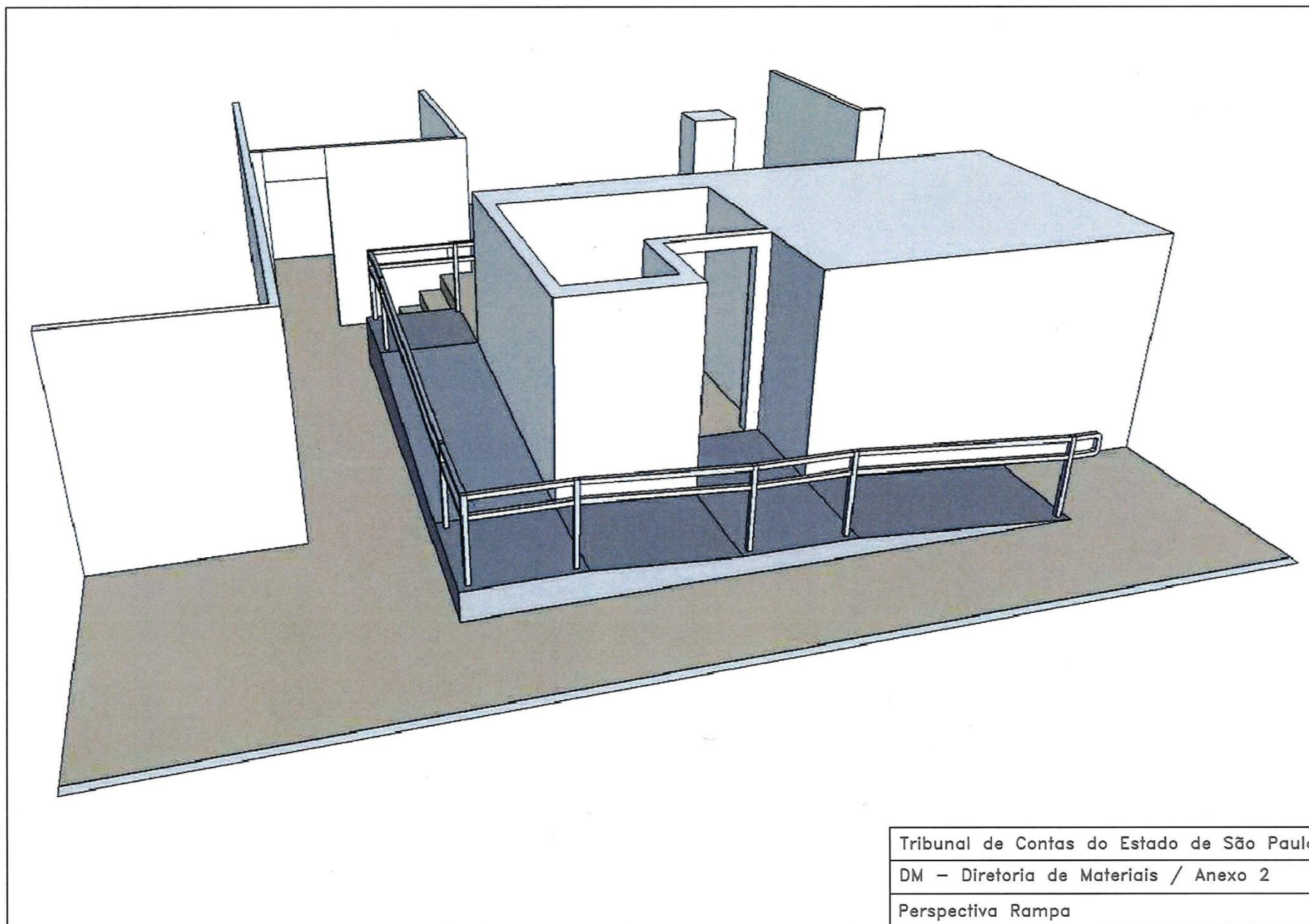
DESENHO 10
