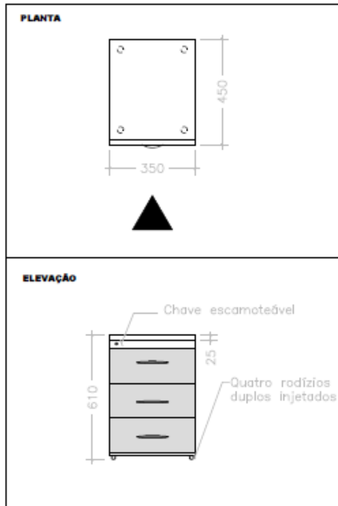
GV Gaveteiro Volante
