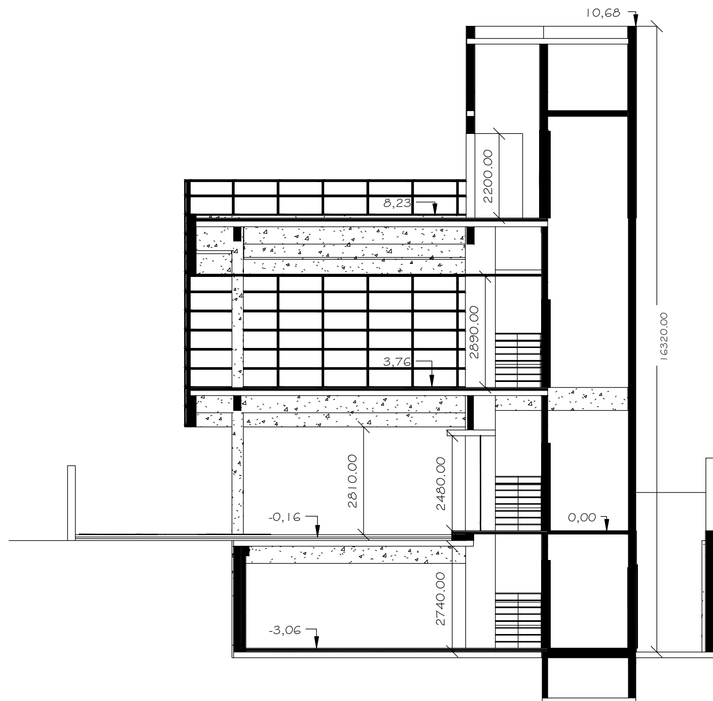
Corte BB
