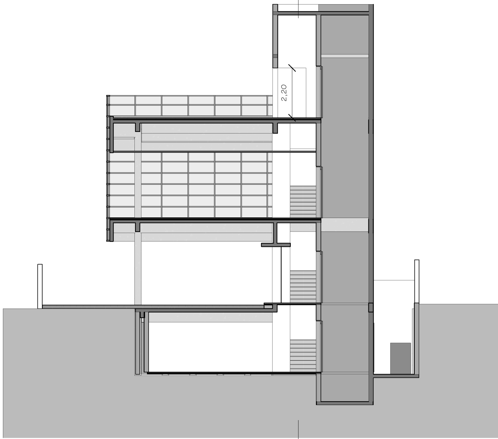
Corte AA 1 : 100
