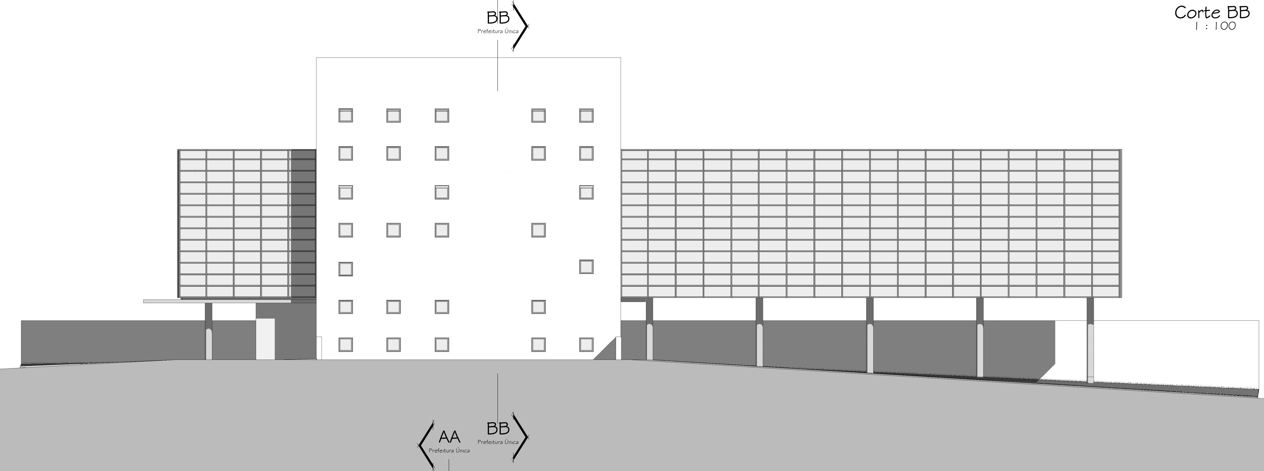
Elevação Direita 1 : 100
