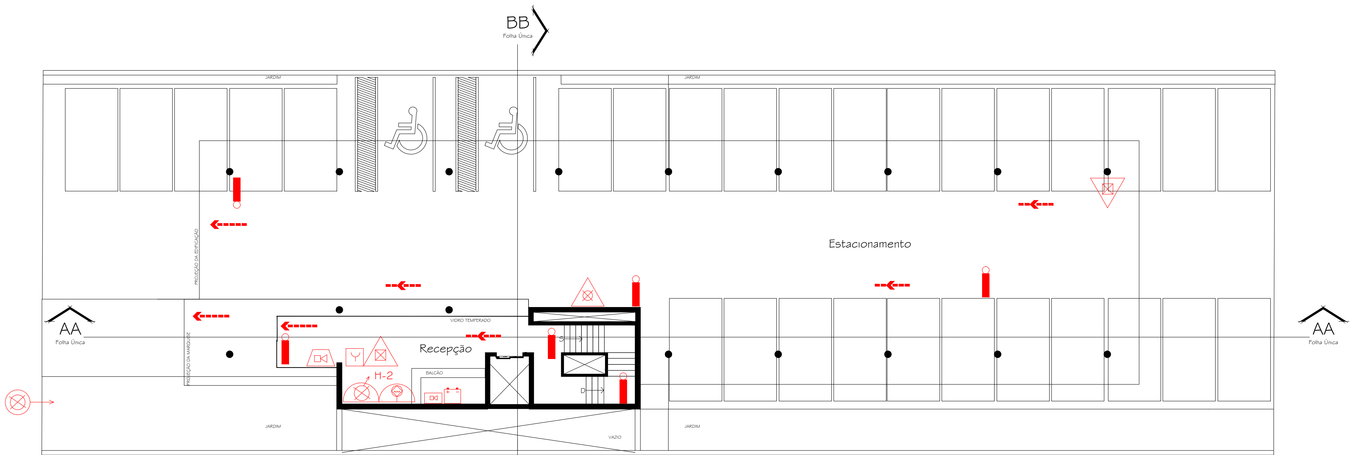
Piso Térreo
