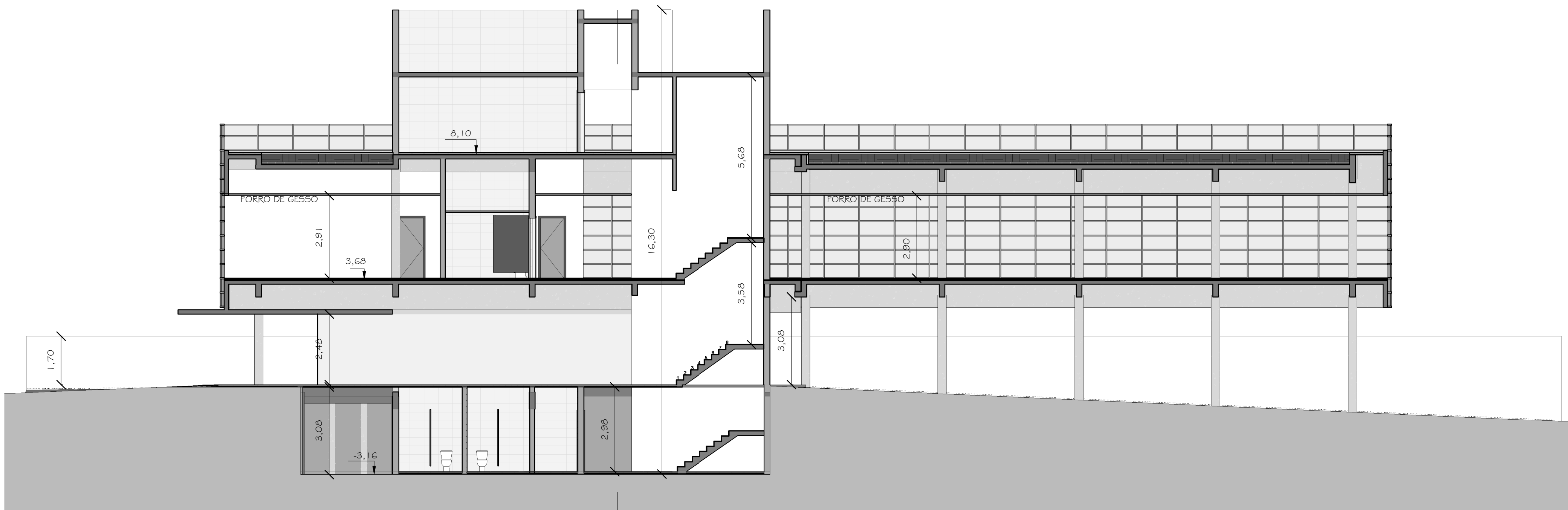
Corte BB 1 : 100
