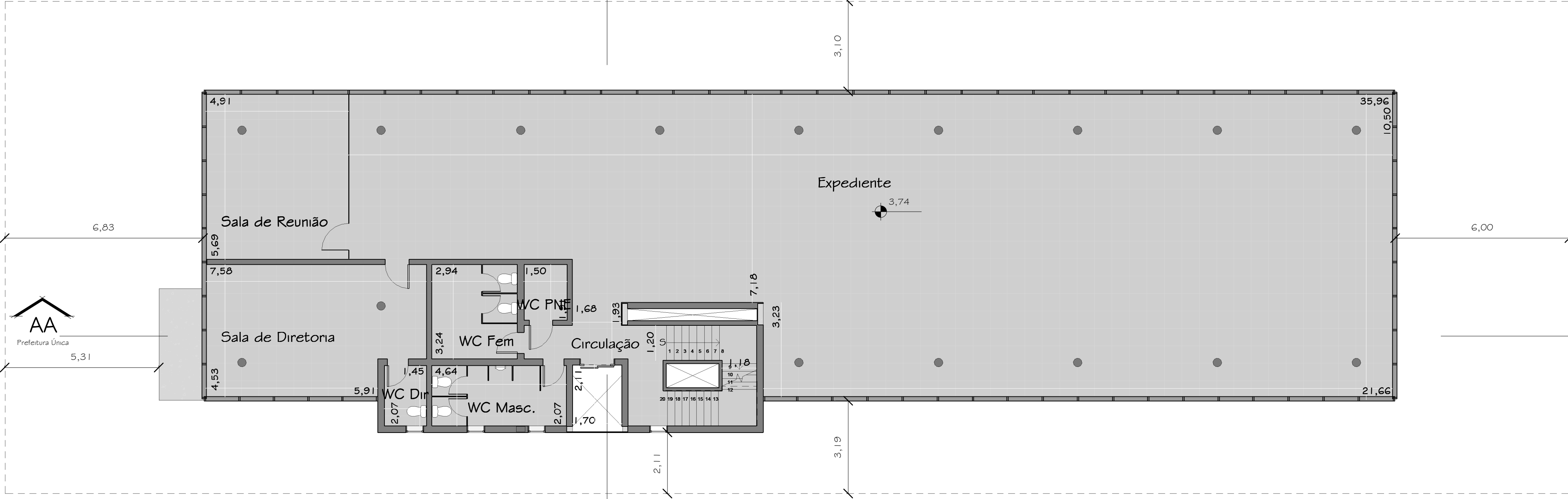
Pavimento Superior 1 : 100
