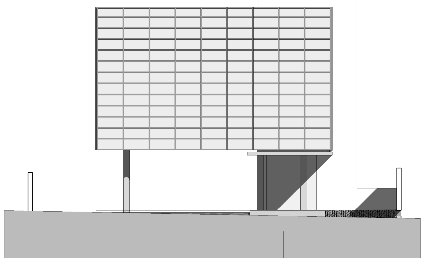
Elevação Anterior 1 : 100
