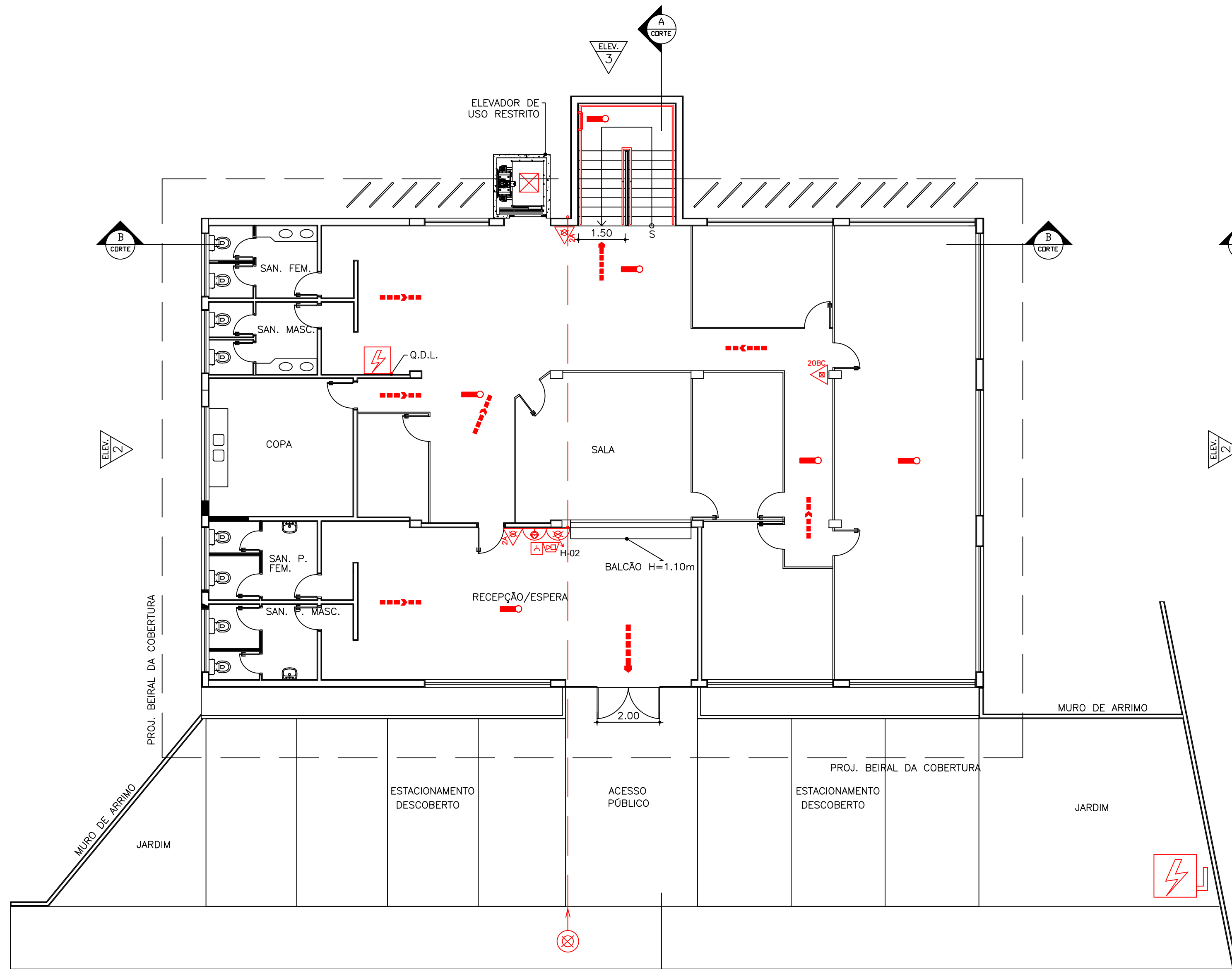
PLANTA PAV. TÉRREO ESCALA 1:100
