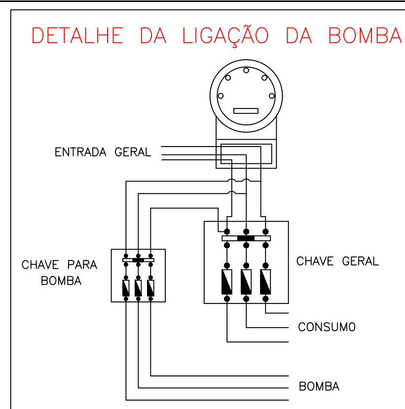
DETALHE DE LIGAÇÃO INDEPENDENTE DA BOMBA ESCALA: SEM ESCALA
