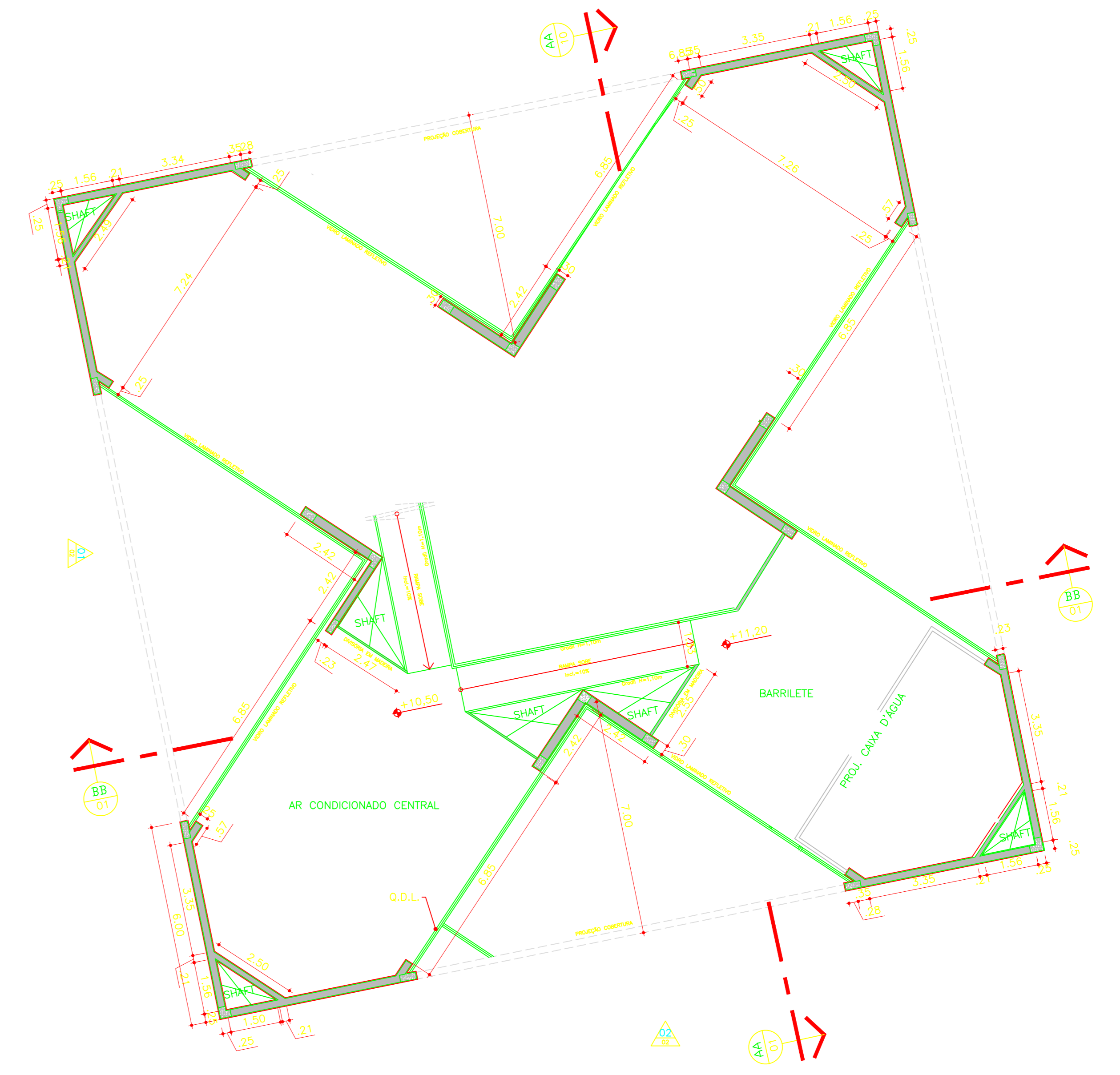
05 PLANTA BARRILETE 1/100
