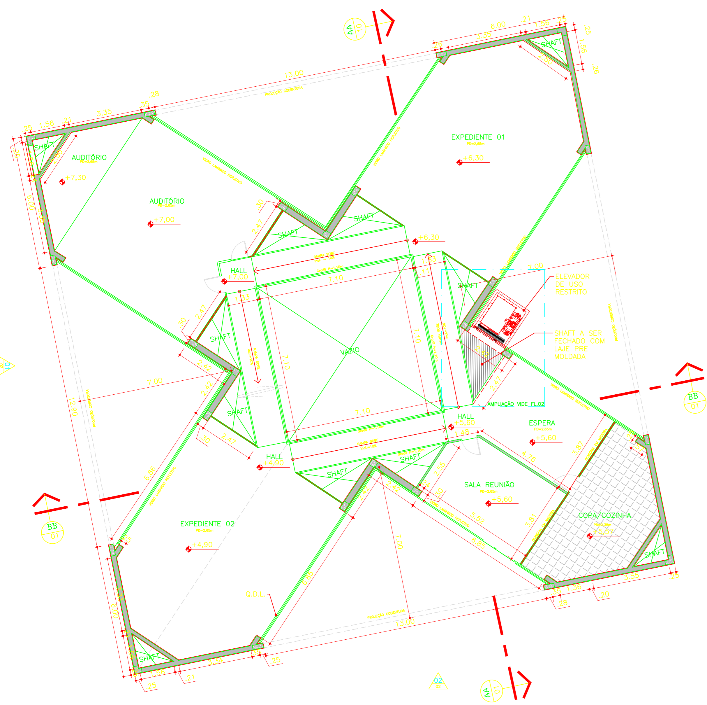
03 PLANTA 1º PAVIMENTO 1/100
