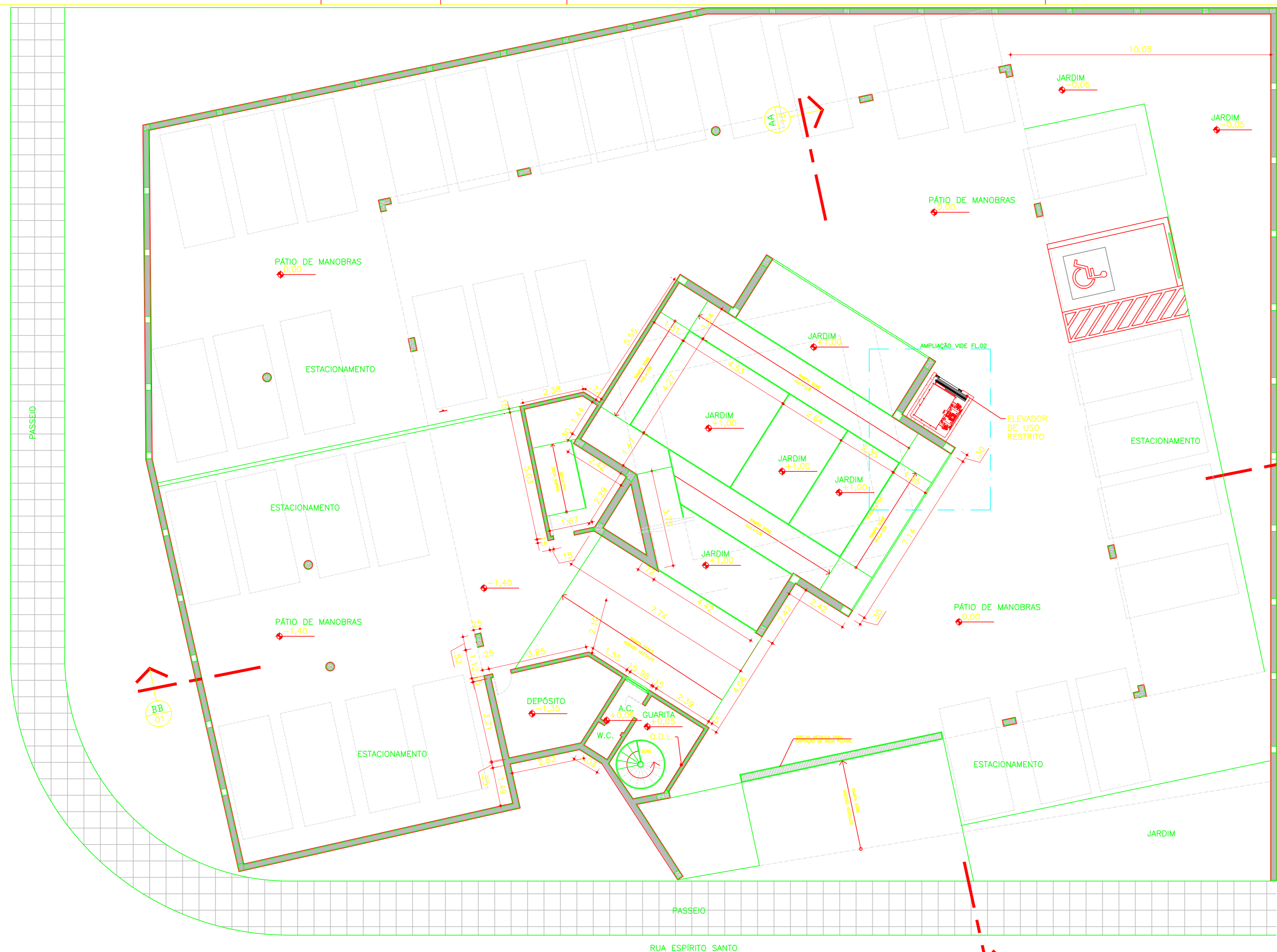
01 PLANTA SUBSOLO 1/100
