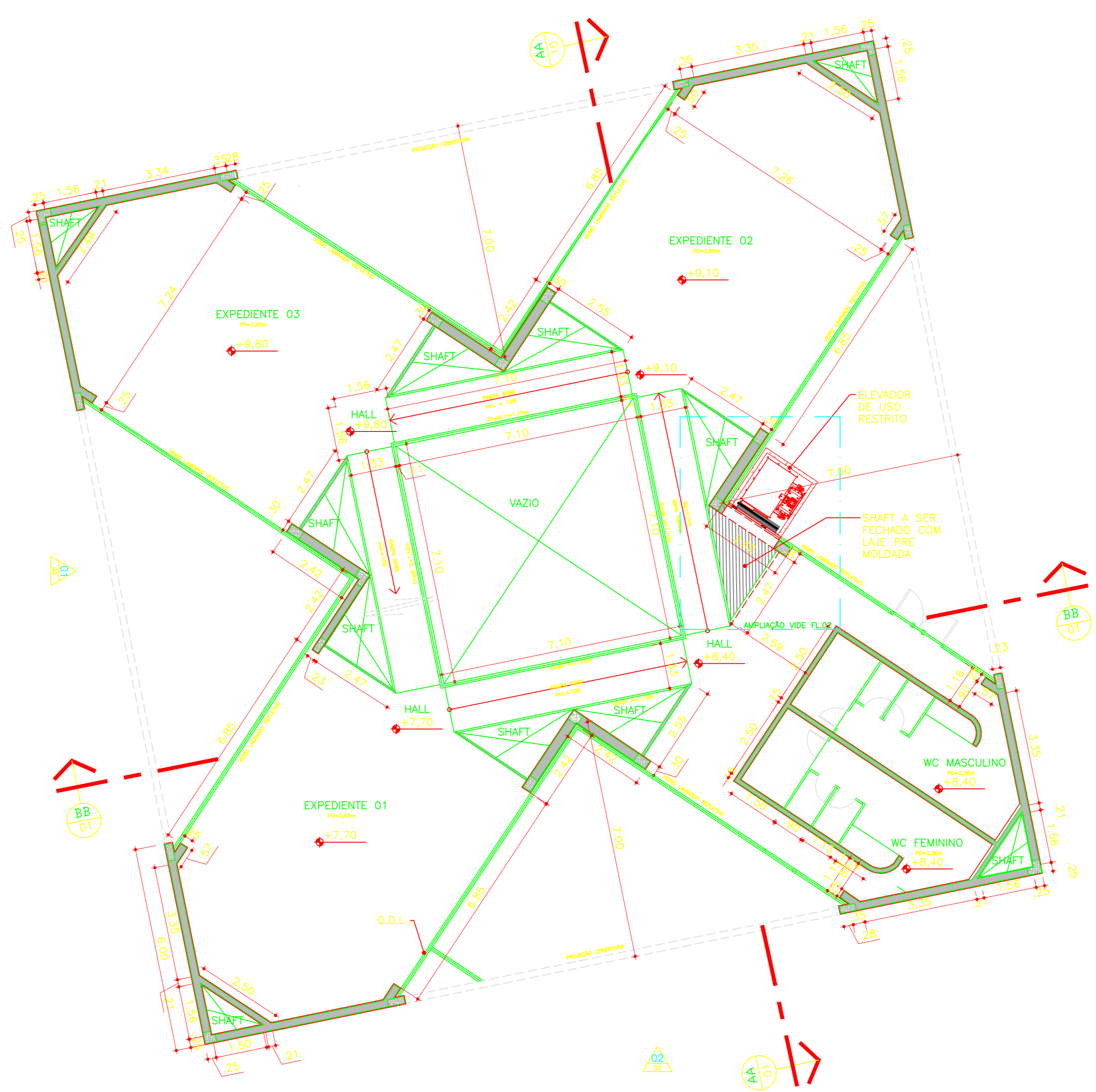
04 PLANTA 2º PAVIMENTO 1/100
