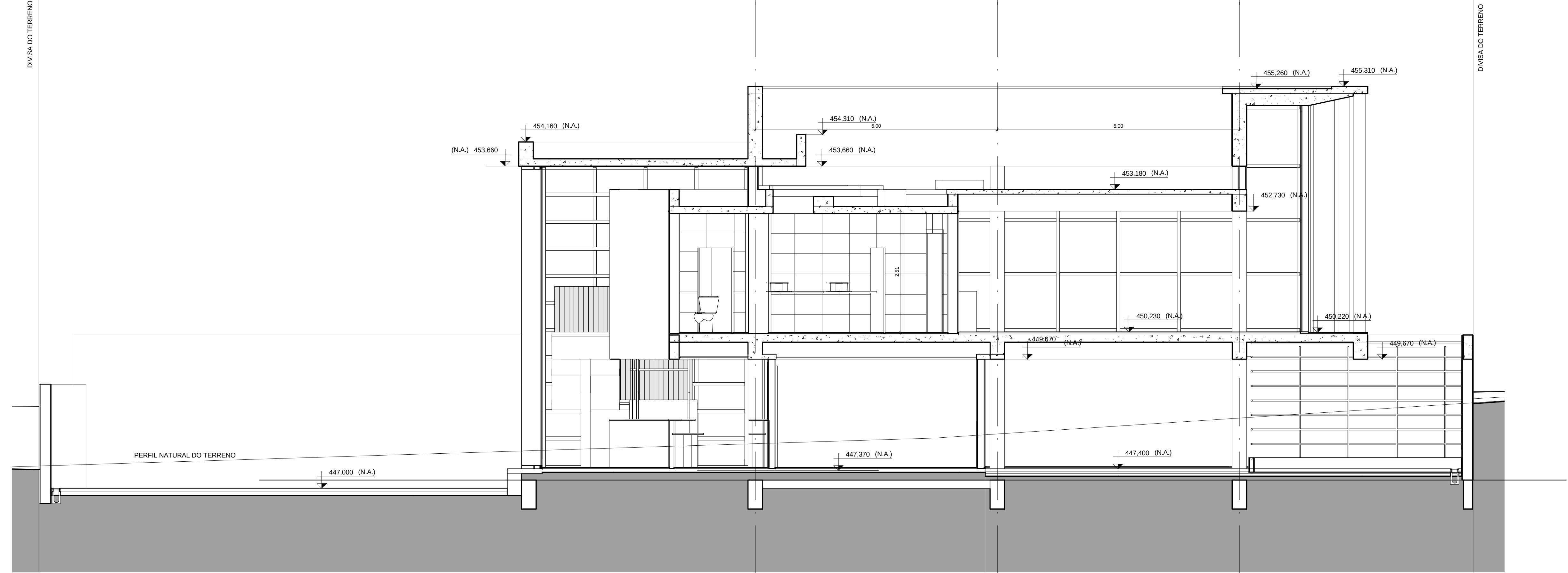
Corte BB 1 : 50
