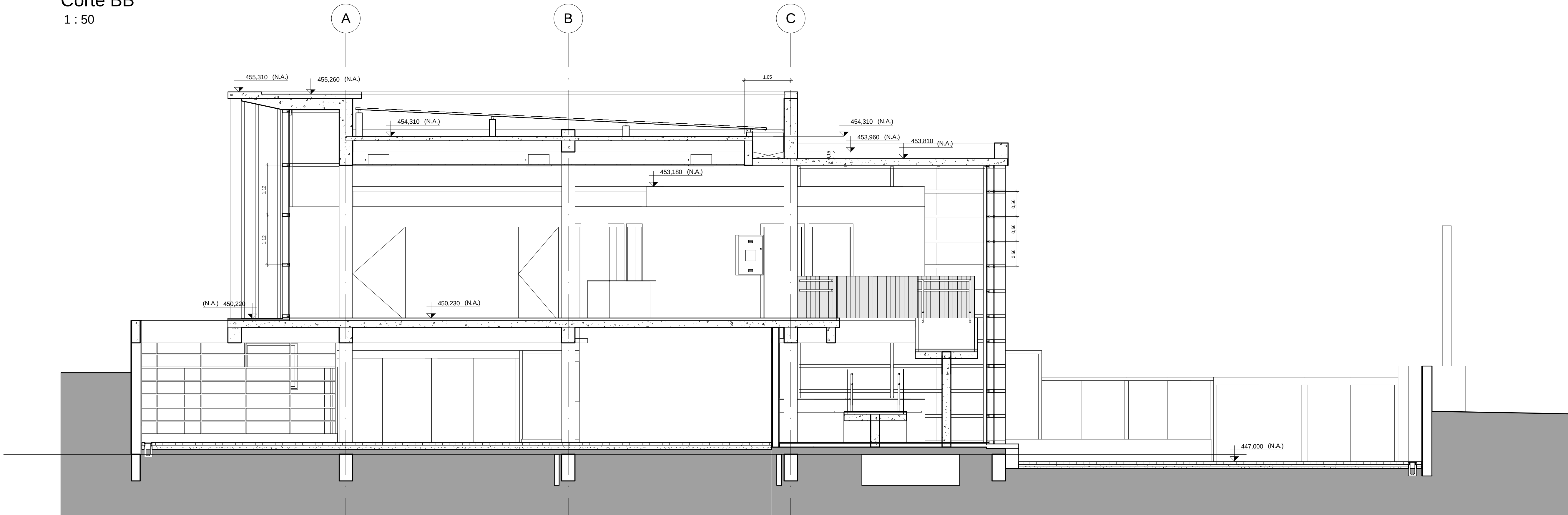
CORTE CC 1 : 50
