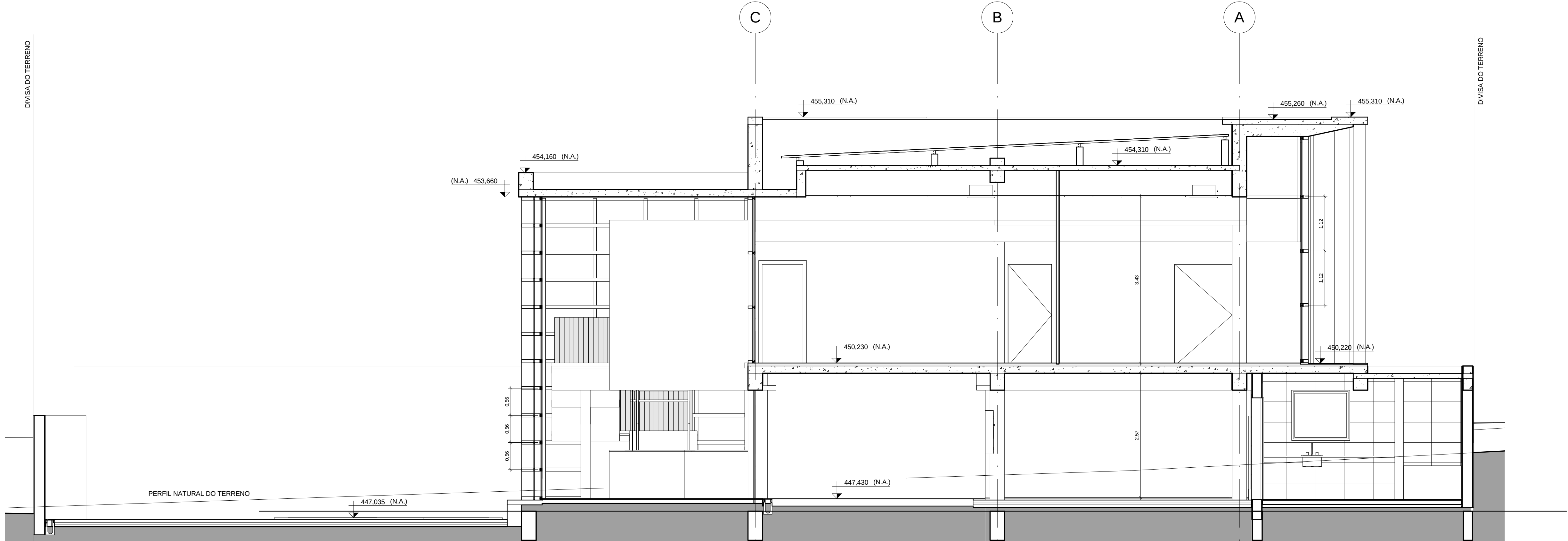
Corte AA 1 : 50
