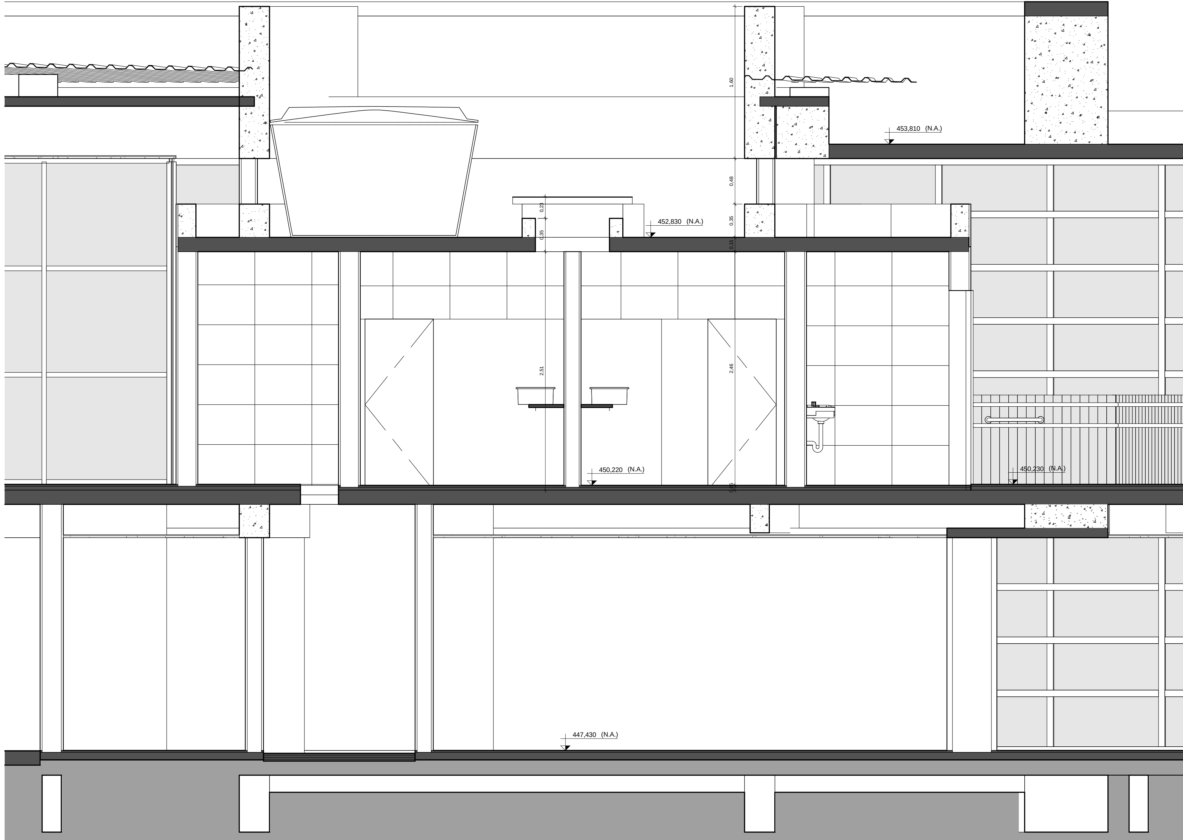
CORTE PARCIAL FF 1 : 25
