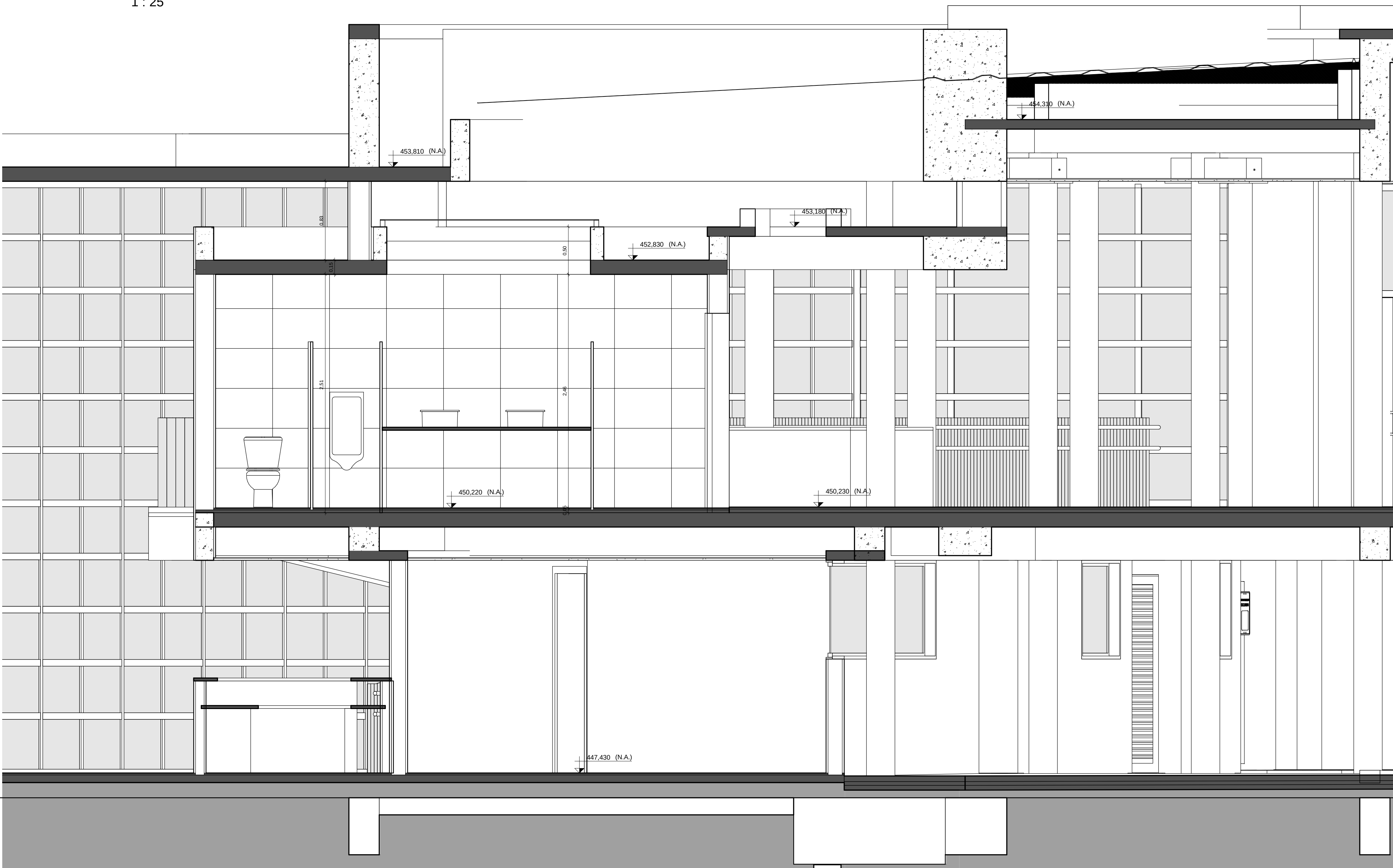
CORTE PARCIAL GG 1 : 25
