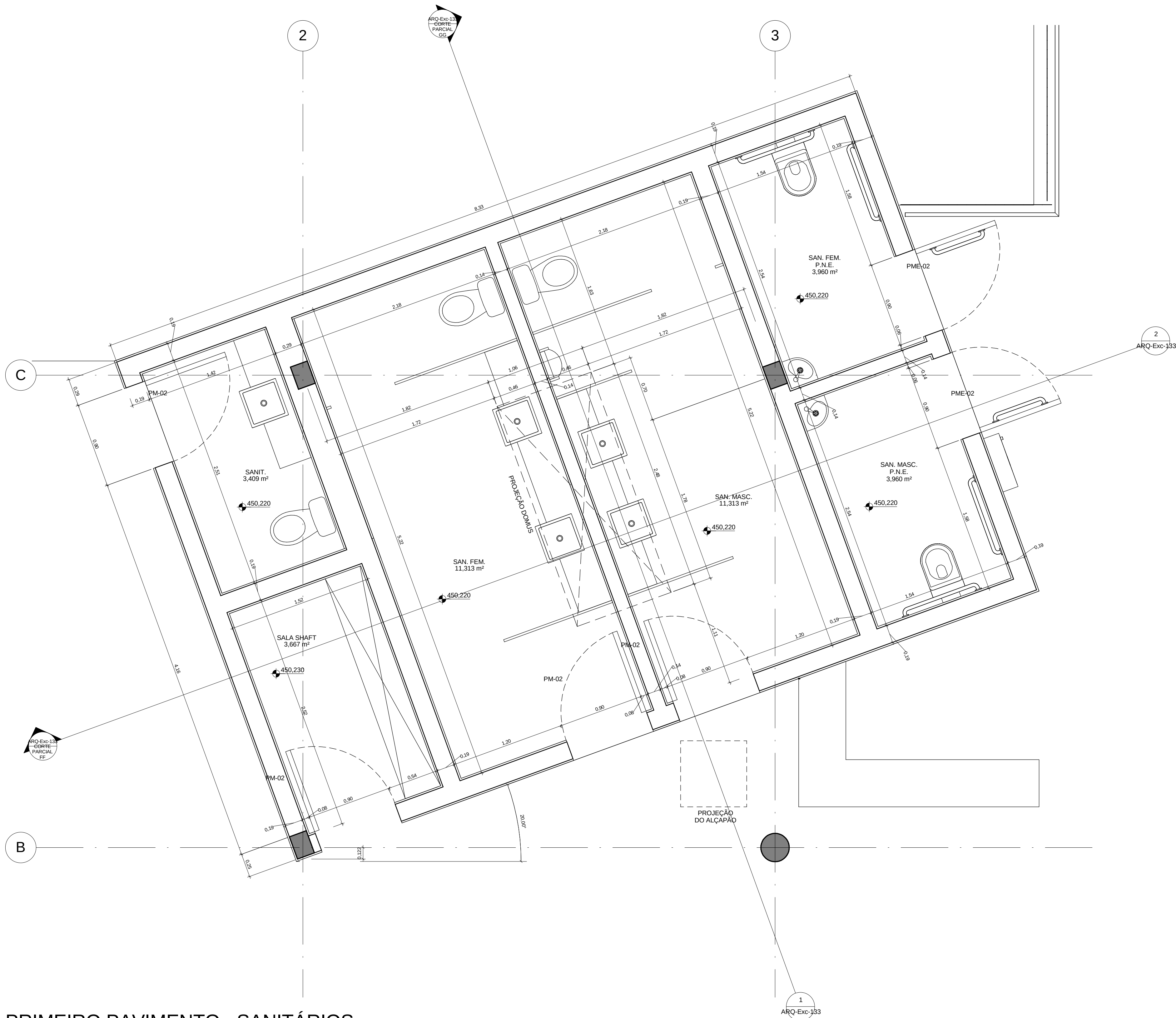
PRIMEIRO PAVIMENTO - SANITÁRIOS 1 : 25
