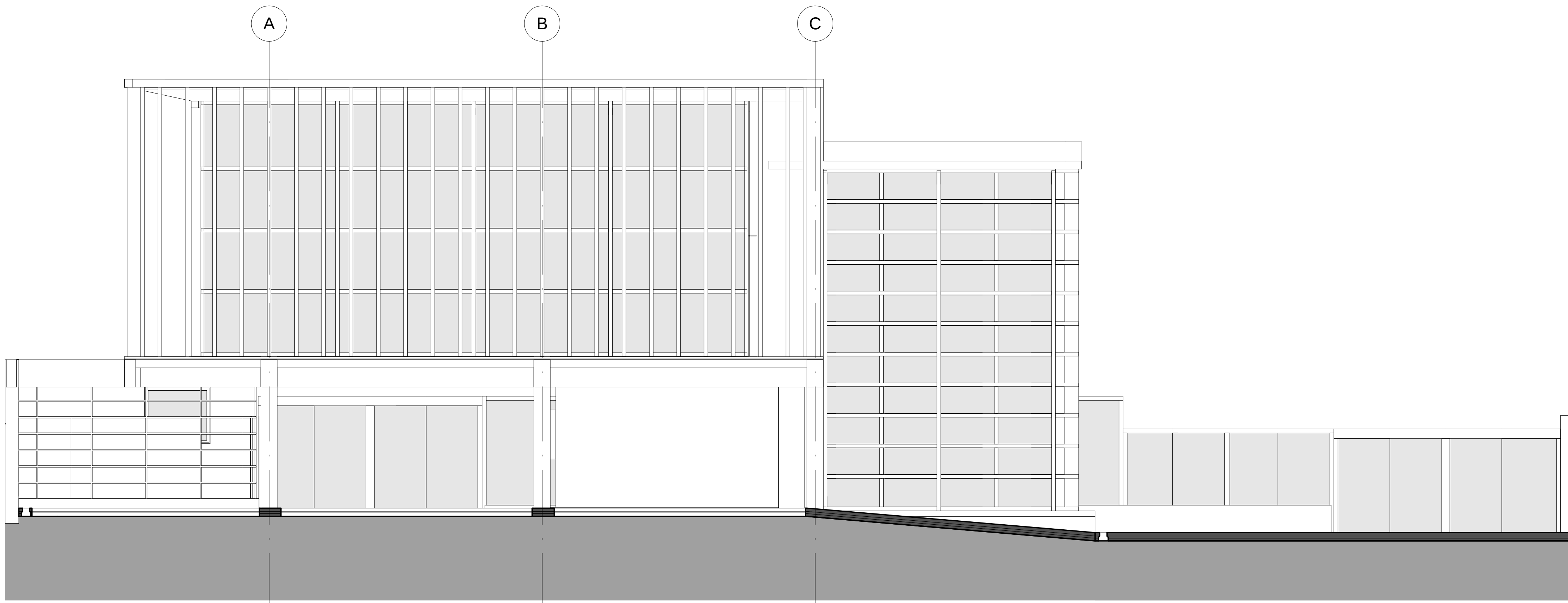
ELEV. NORDESTE 1 : 50
