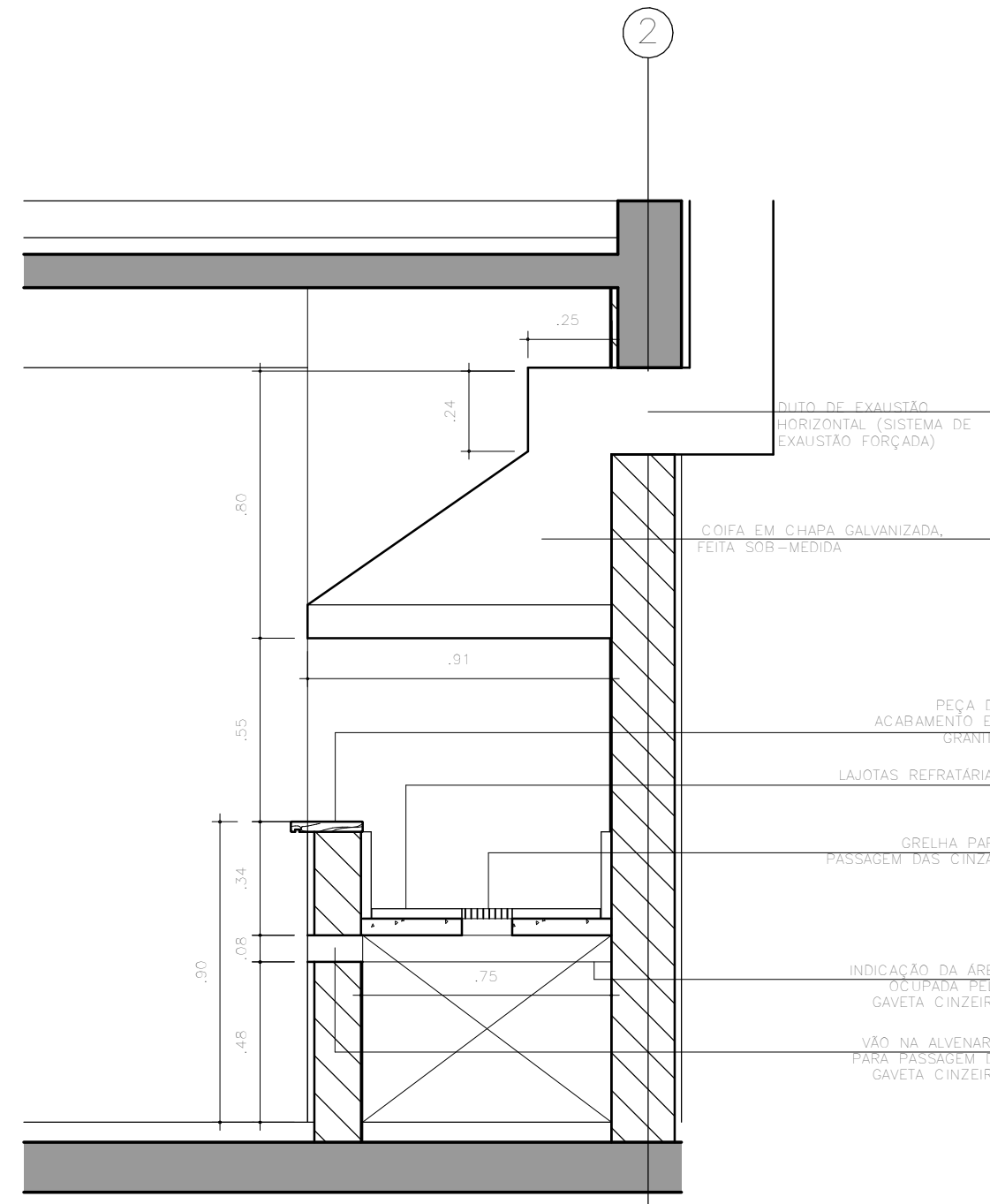
DETALHE 3.3.1 - ESTRUTURA PARA EMBUTIR CHURRASQUEIRA ÁREAS MOLHADAS - COPA/COZINHA - PAVIMENTO TERREO CORTE ESC. 1:20
