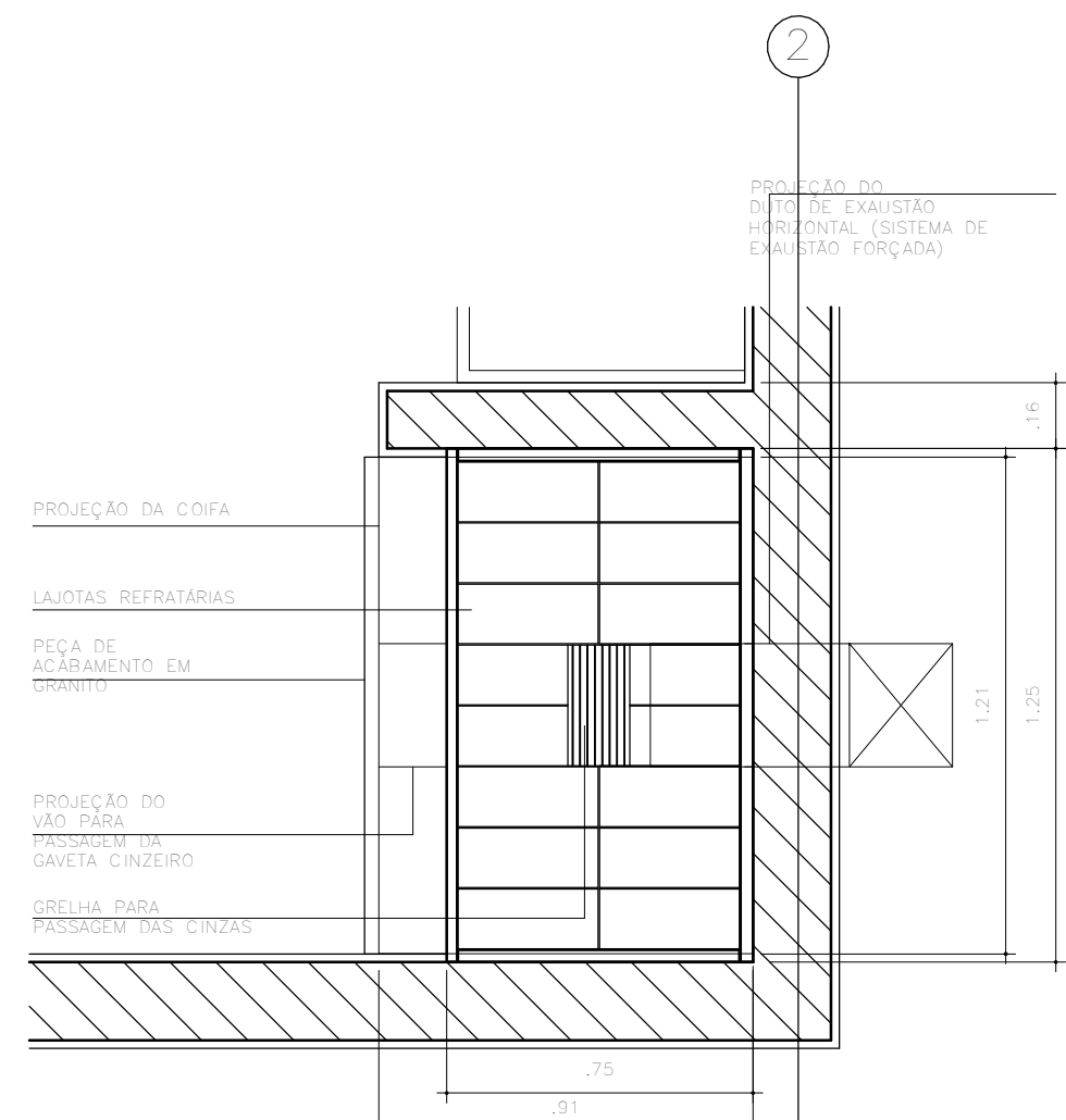
DETALHE 3.3.1 - ESTRUTURA PARA EMBUTIR CHURRASQUEIRA ÁREAS MOLHADAS - COPA/COZINHA - PAVIMENTO TERREO PLANTA ESC. 1:20
