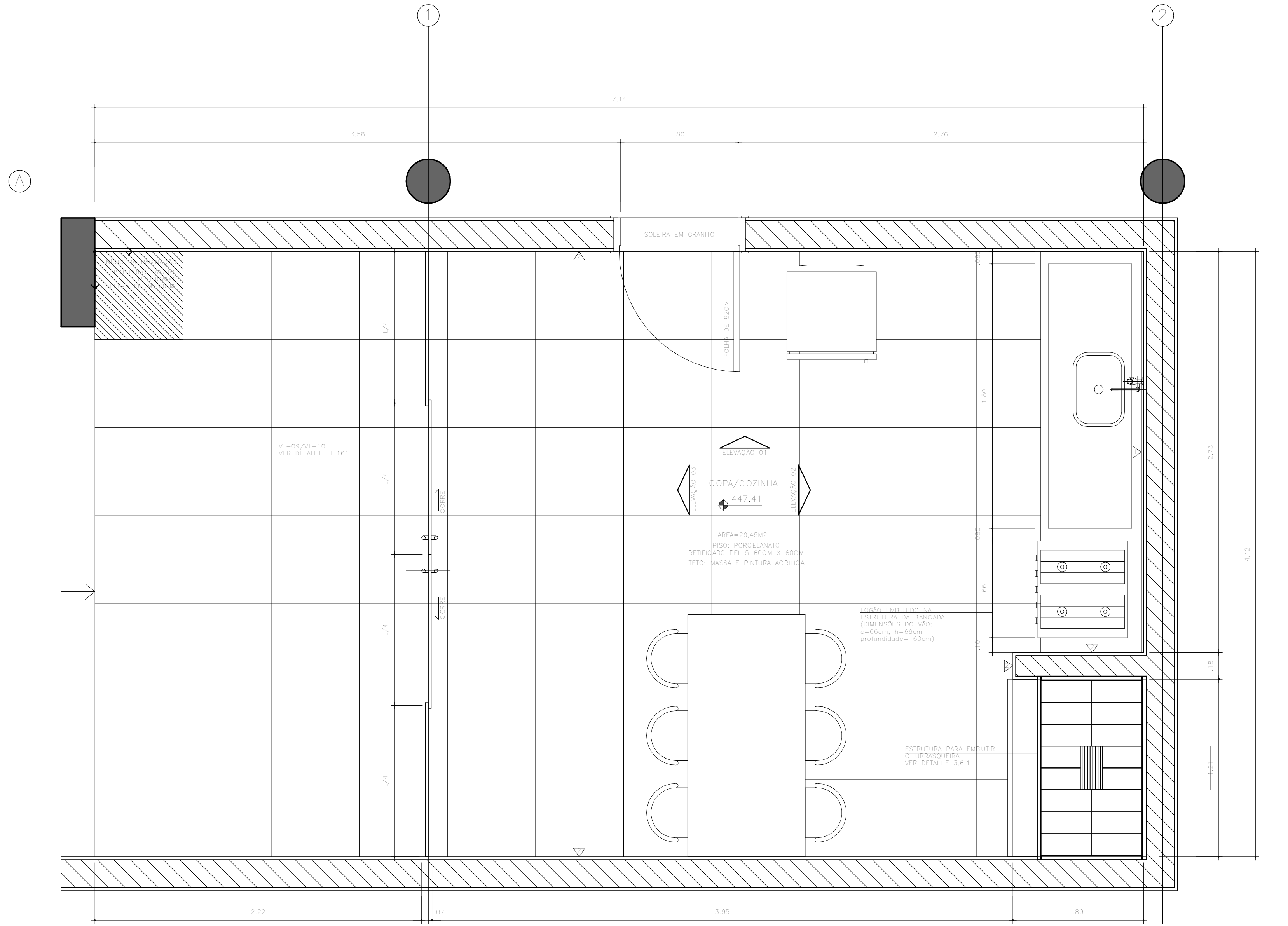
DETALHE 3.3 ÁREAS MOLHADAS - COPA/COZINHA - PAVIMENTO TERREO PLANTA ESC. 1:20
