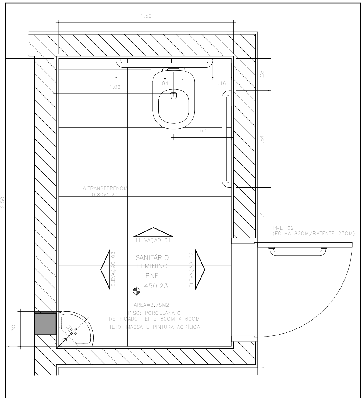
DETALHE 3.5 - ÁREAS MOLHADAS SANITÁRIO FEM/MASC PNE - PRIMEIRO PAVIMENTO ESC. 1:20
