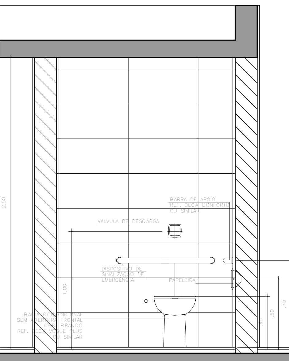
DETALHE 3.5 - ÁREAS MOLHADAS SANITÁRIO FEM/MASC PNE - PRIMEIRO PAVIMENTO ELEVÇÃO 01 ESC. 1:20
