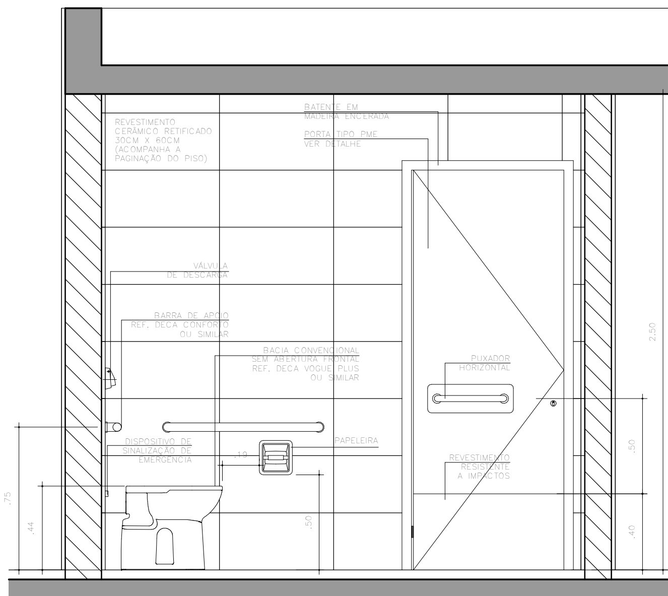
DETALHE 3.5 - ÁREAS MOLHADAS SANITÁRIO FEM/MASC PNE - PRIMEIRO PAVIMENTO ELEVÇÃO 02 ESC. 1:20
