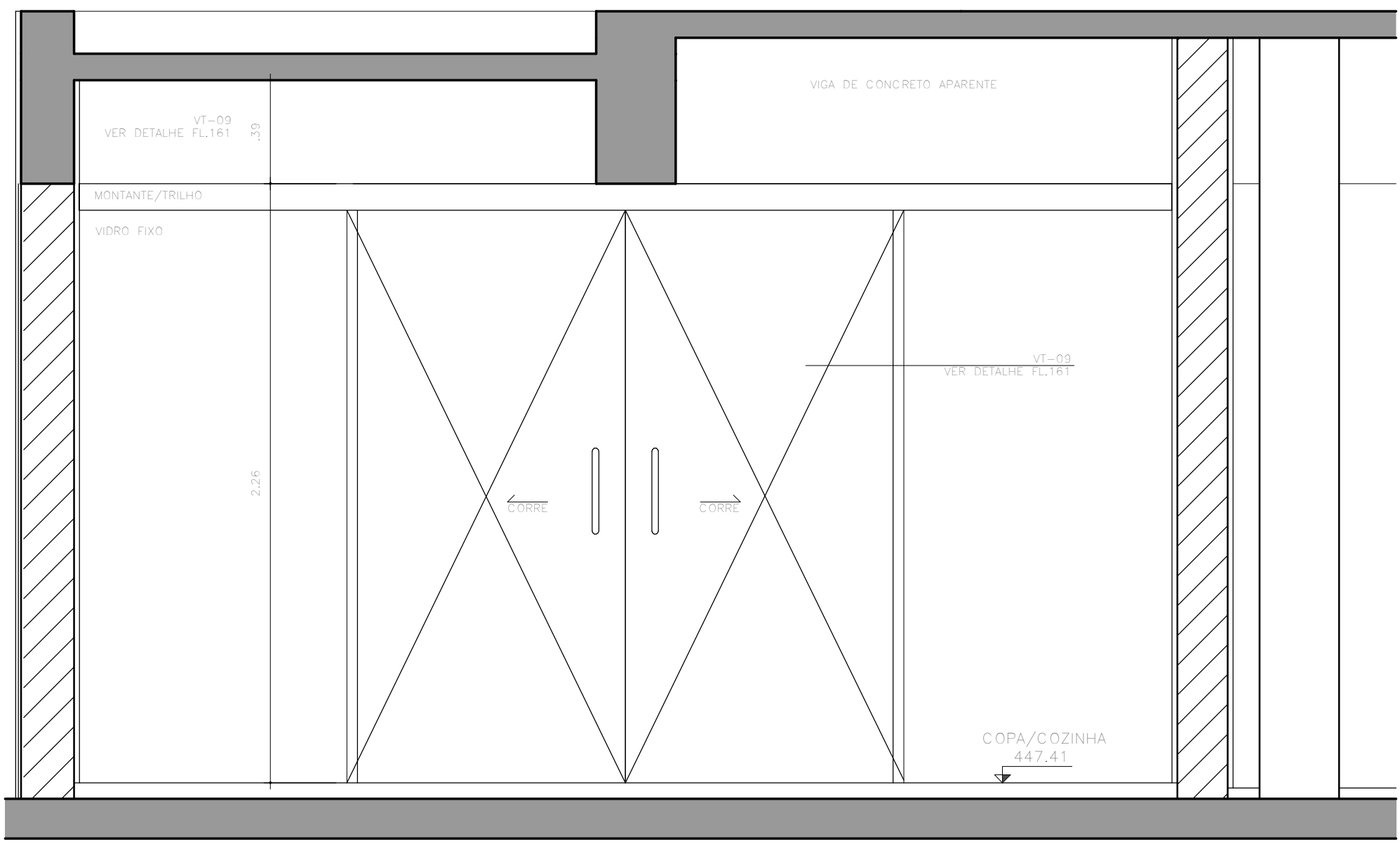
DETALHE 3.3 ÁREAS MOLHADAS - COPA/COZINHA - PAVIMENTO TERREO ELEVÇÃO 03 ESC. 1:20
