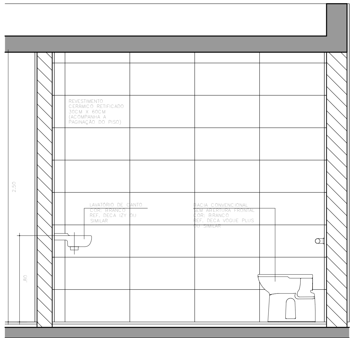
DETALHE 3.5 - ÁREAS MOLHADAS SANITÁRIO FEM/MASC PNE - PRIMEIRO PAVIMENTO ELEVÇÃO 03 ESC. 1:20
