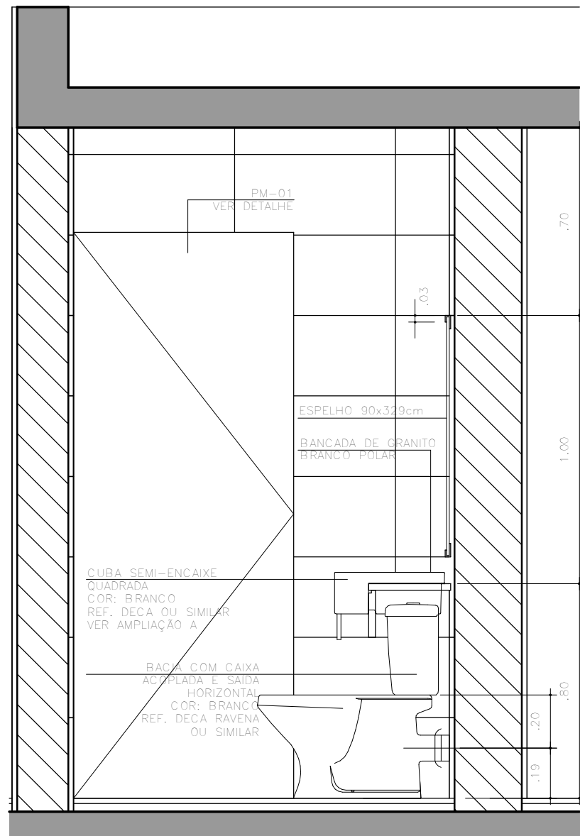
DETALHE 3.4 - ÁREAS MOLHADAS SANITÁRIO DIREÇÃO - PRIMEIRO PAVIMENTO ELEVÇÃO 01 ESC. 1:20
