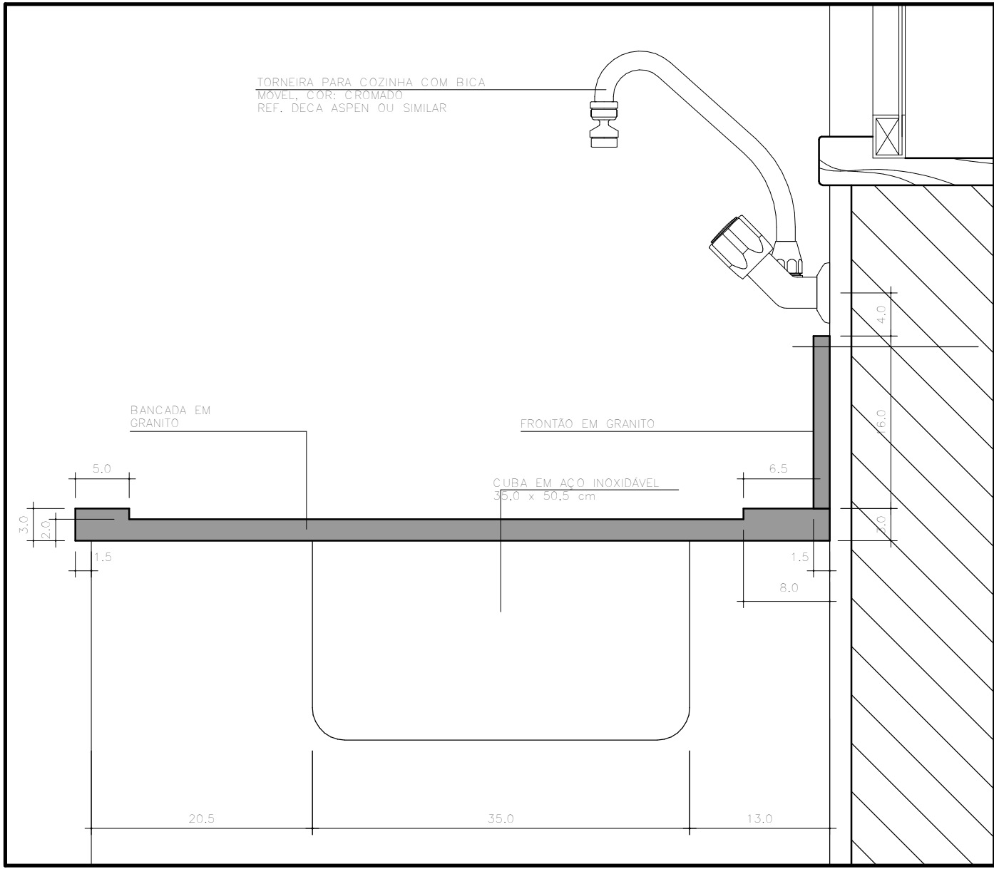
DETALHE 3.3 AMPLIAÇÃO A - BANCADA DE GRANITO medidos em cm ESC. 1:5
