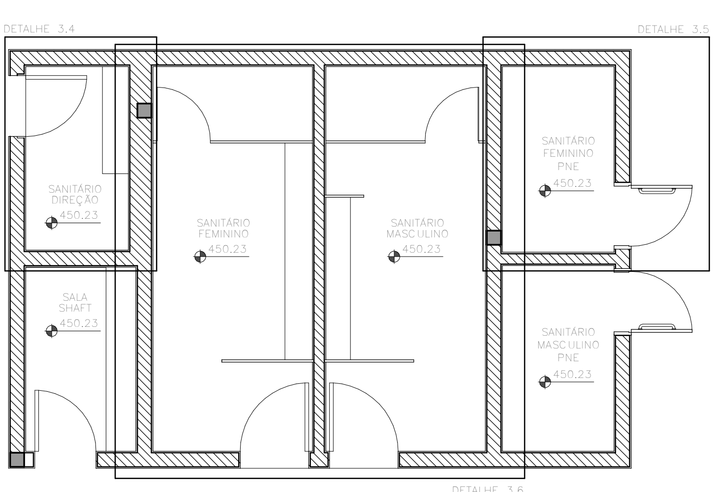
ÁREAS MOLHADAS - PRIMEIRO PAVIMENTO - INDICAÇÃO DE DETALHES PLANTA SEM ESCALA
