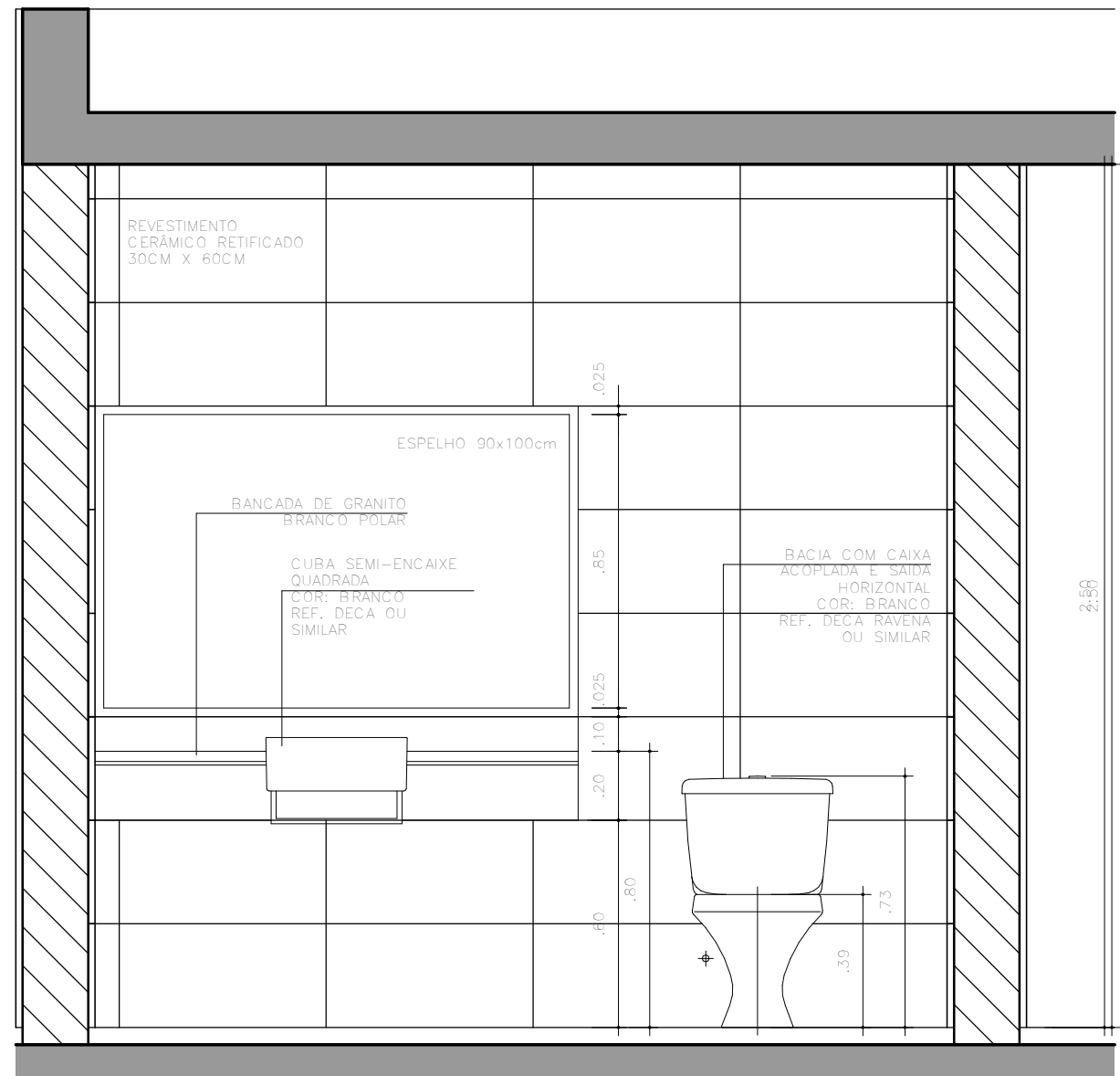
DETALHE 3.4 - ÁREAS MOLHADAS SANITÁRIO DIREÇÃO - PRIMEIRO PAVIMENTO ELEVÇÃO 02 ESC. 1:20
