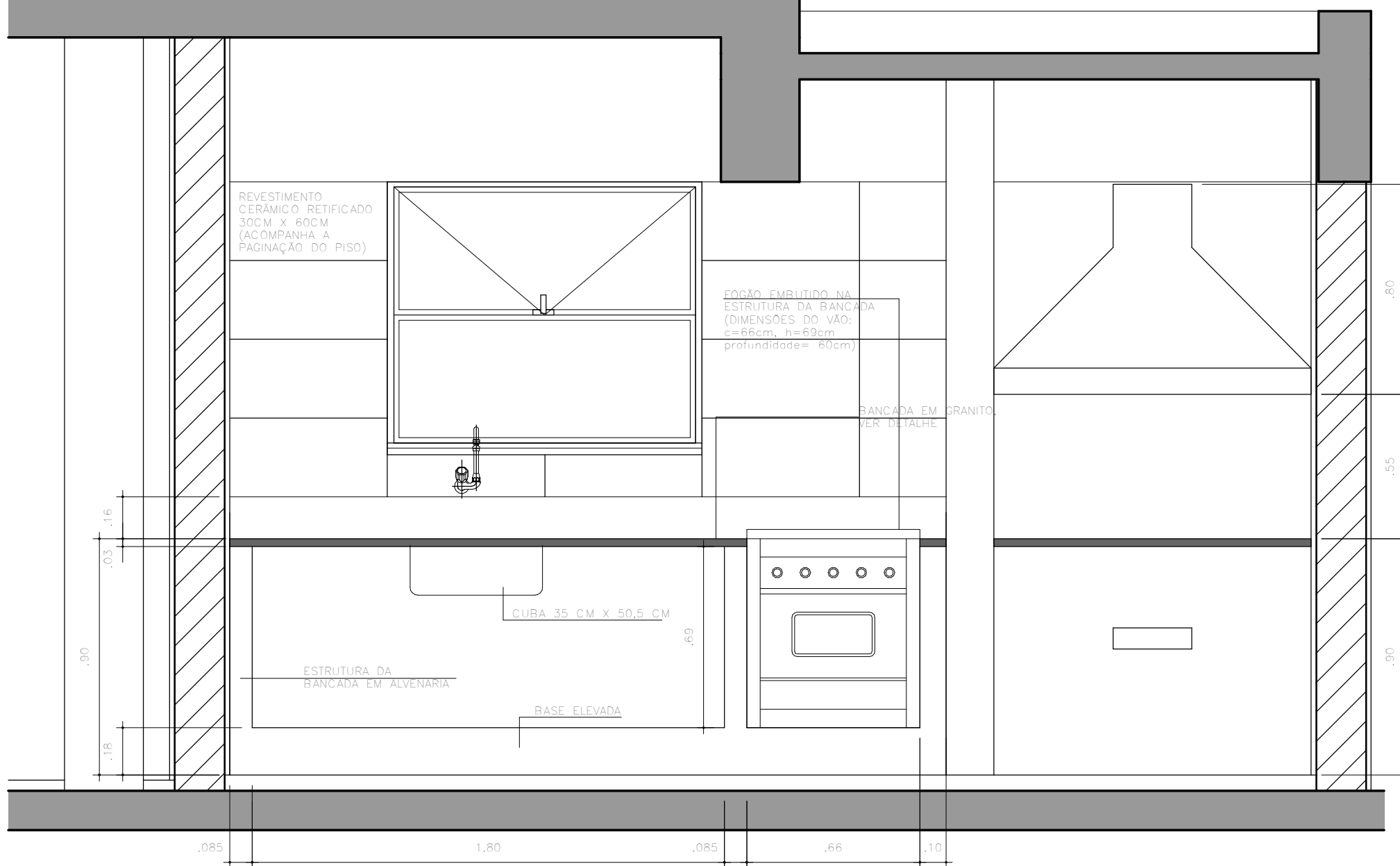
DETALHE 3.3 ÁREAS MOLHADAS - COPA/COZINHA - PAVIMENTO TERREO ELEVÇÃO 02 ESC. 1:20
