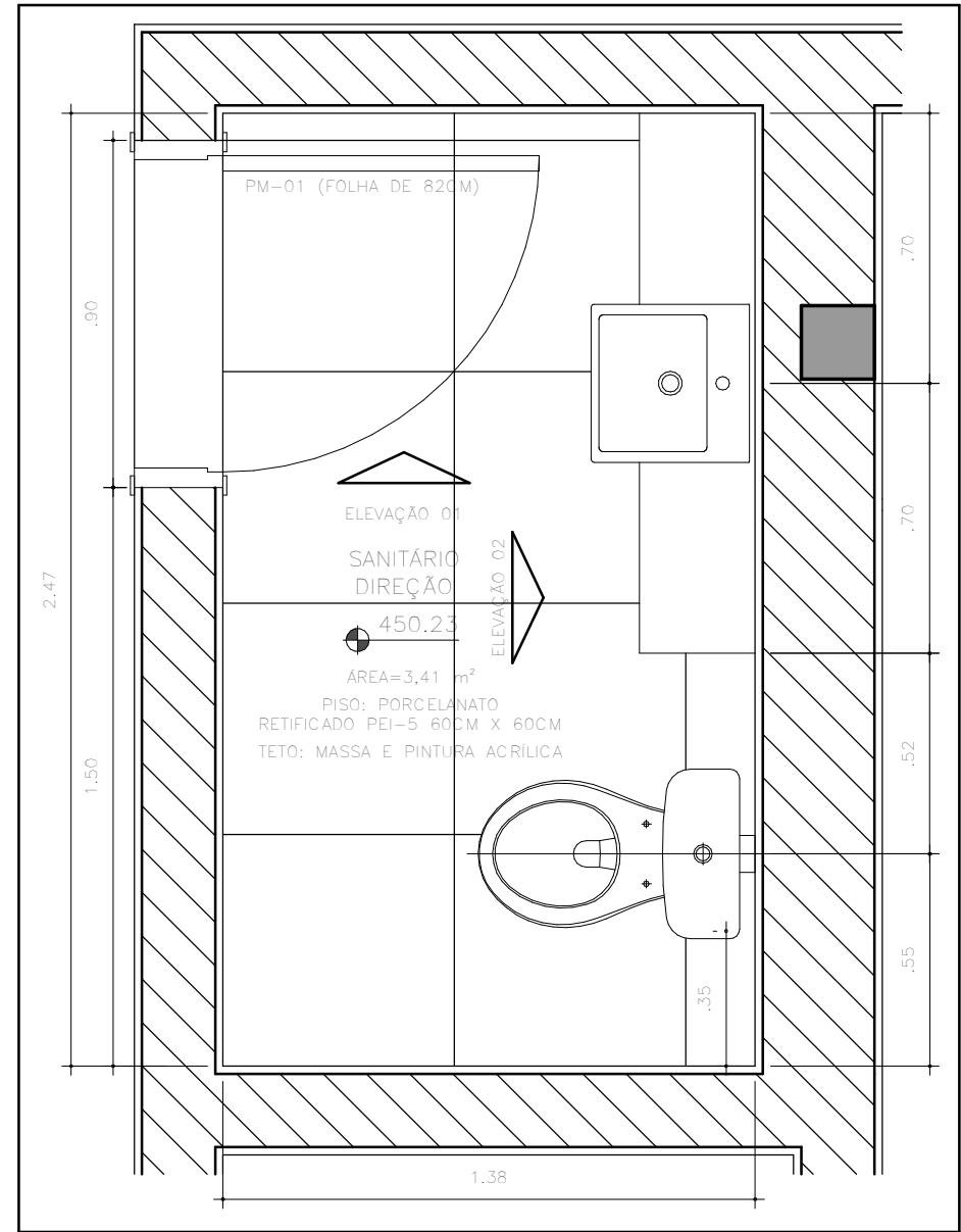
DETALHE 3.4 - ÁREAS MOLHADAS SANITÁRIO DIREÇÃO - PRIMEIRO PAVIMENTO ESC. 1:20
