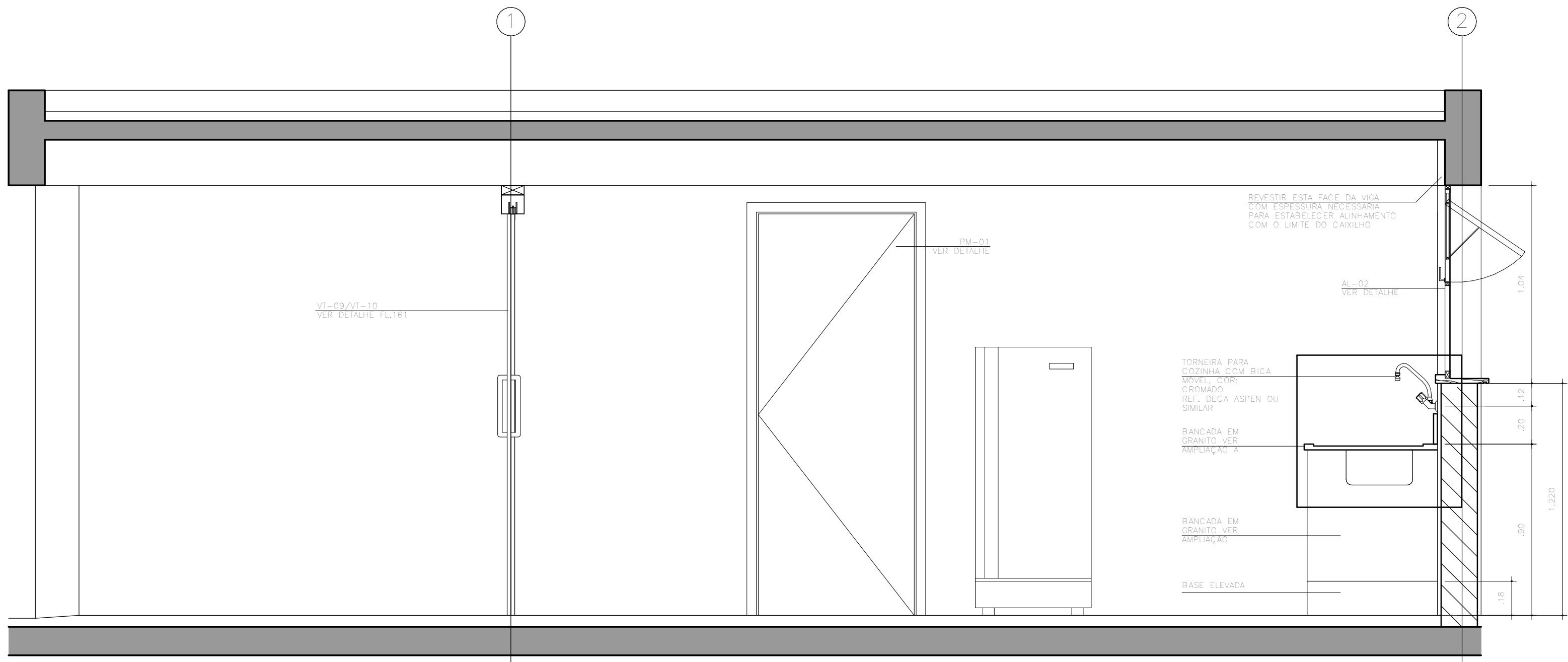
DETALHE 3.3 ÁREAS MOLHADAS - COPA/COZINHA - PAVIMENTO TERREO ELEVÇÃO 01 ESC. 1:20
