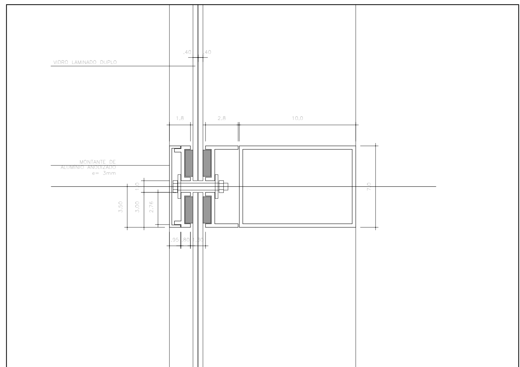
AMPLIAÇÃO A ESC. 1:2
