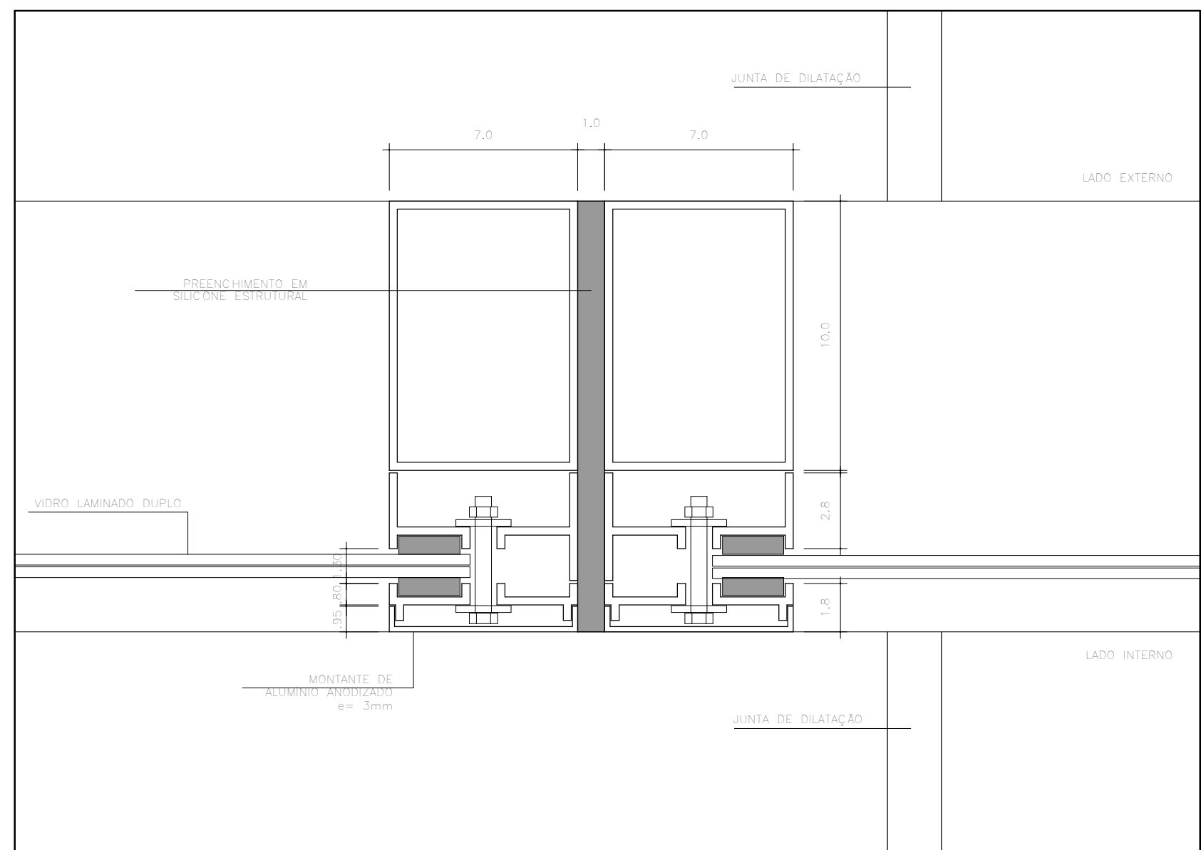
AMPLIAÇÃO B ESC. 1:2
